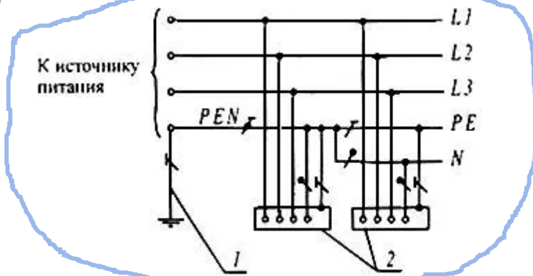
Рис.3. Переходная система TN – C - S переменного тока.
