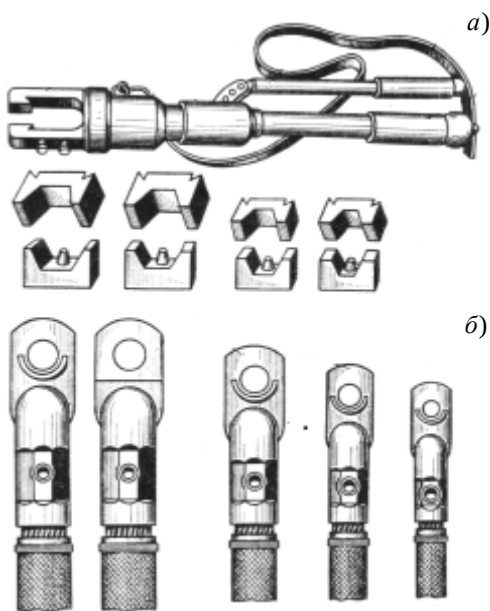
Рисунок 1.1 – Пресс (а) и наконечники (б)
