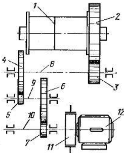
Рис. 2 Кинематическая схема электрической лебёдки: 1 — барабан, 2 - 7 — шестерни редуктора, 8 - 10 — валы редуктора, 11 — тормозное устройство, 12 — электродвигатель.
