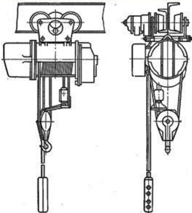
Рис. 3. Электрическая таль типа ТЭ
