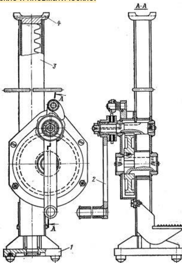
Рис. 1. Реечный домкрат
