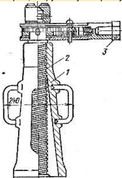
Рис. 2. Винтовой домкрат
