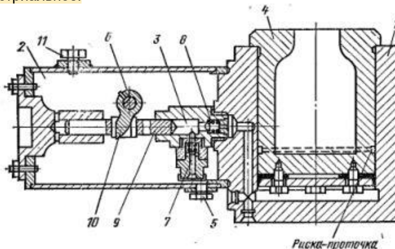
Рис. 3. Гидравлический домкрат
