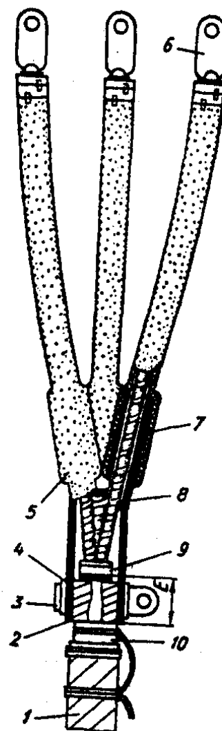
Рис. 7.31. Концевая заделка типа КВР в резиновой перчатке:
