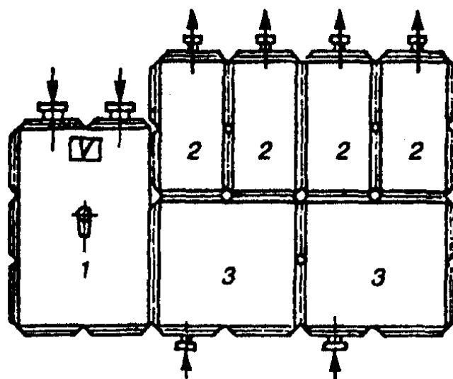
Рис. 6.4. Сборное распределительное устройство РУС-Е:
