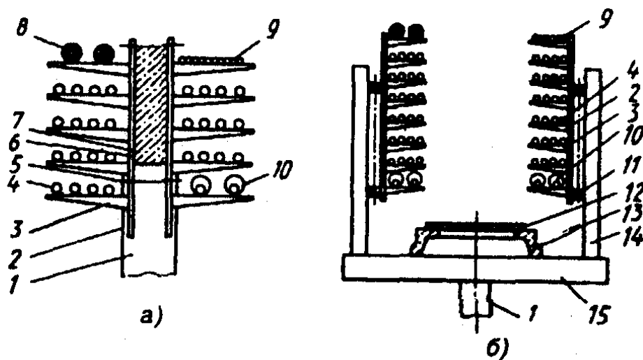
Рис. 7.8. Прокладка кабелей на эстакадах:
