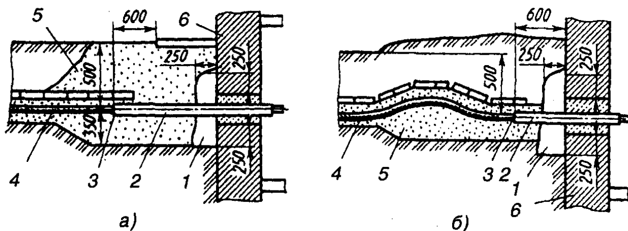
Рис. 7.4. Ввод кабелей из траншеи в здание или кабельное сооружение:
