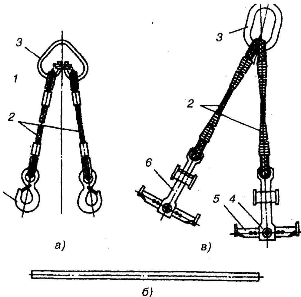
Рис. 7.11. Грузозахватные приспособления:
