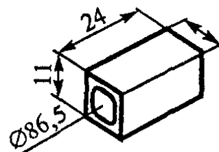
Рис. 1.21. Бирки маркировочные БМП-4
