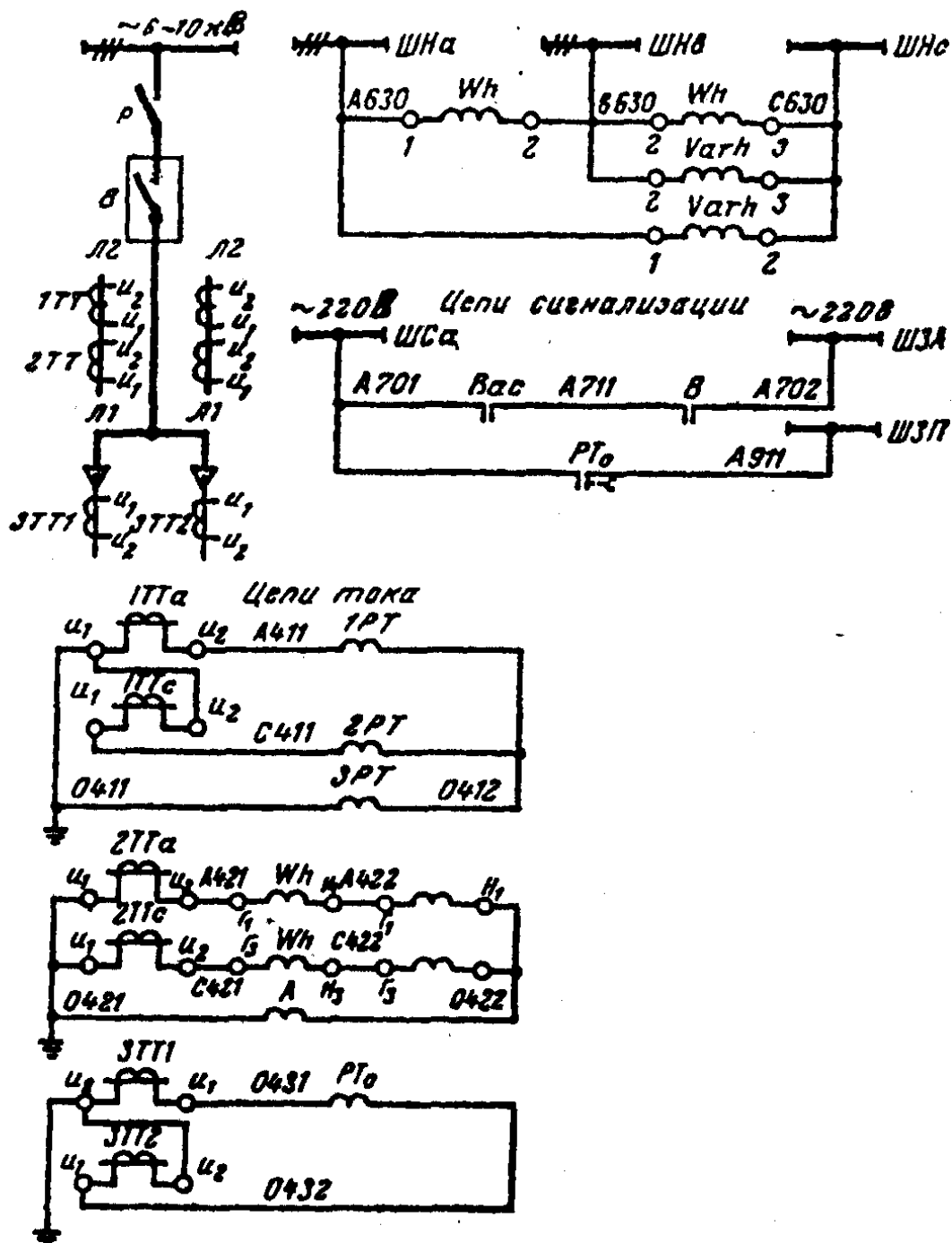
Рис. 1.4. Принципиальная схема управления и защиты присоединения 6—10 кВ
