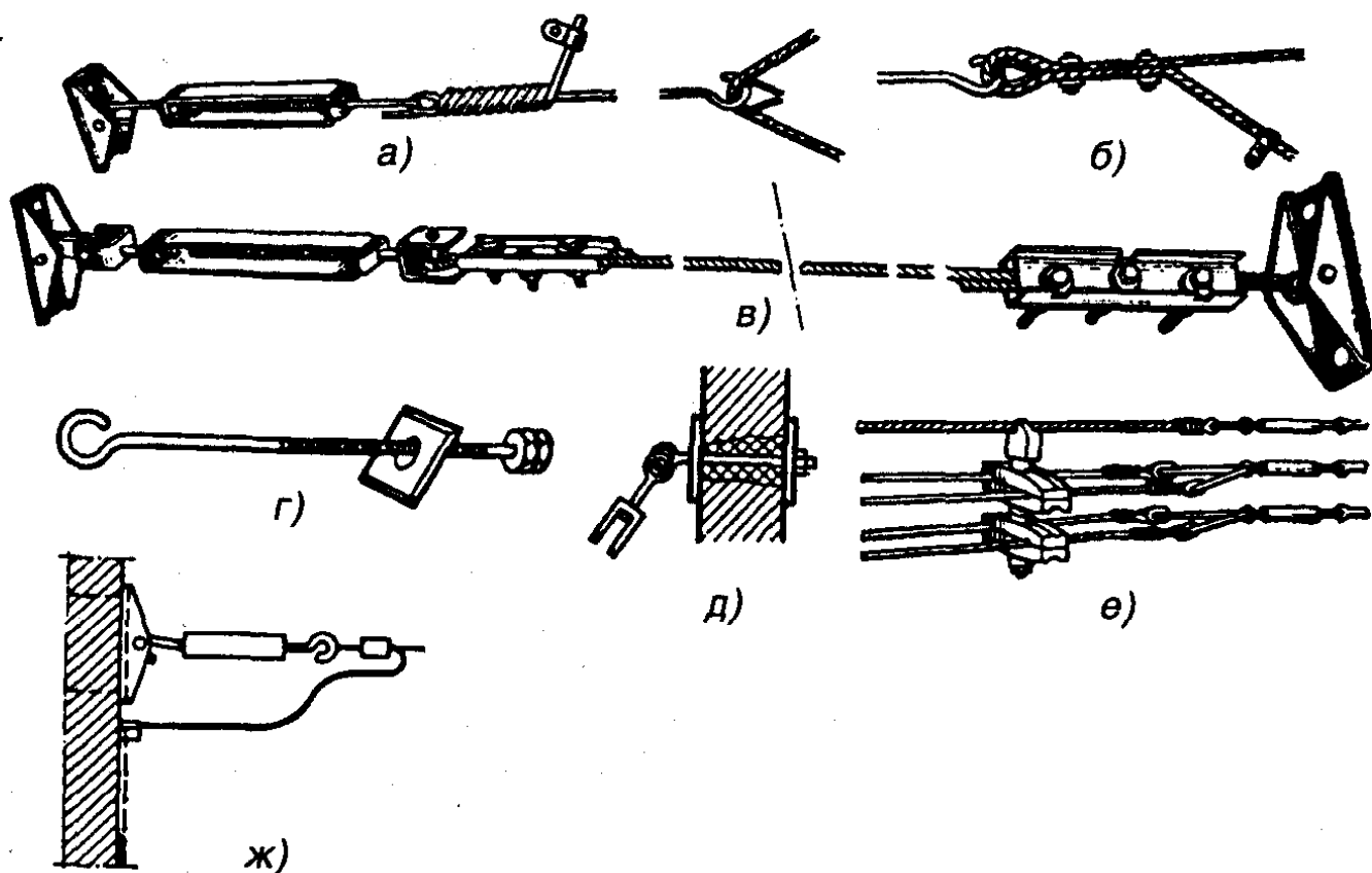
Рис. 4.6. Монтаж элементов тросовых электропроводок:
