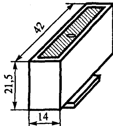
Рис. 1.18. Колодки маркировочные типа КМ
