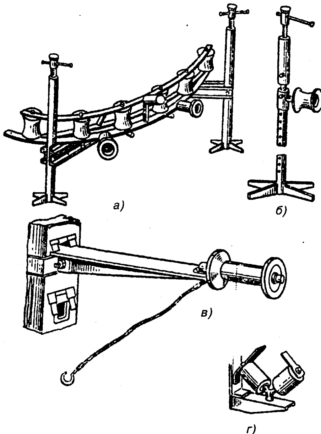
Рис. 7.13. Приспособление для раскатки кабеля: а — угловой универсальный ролик; б — г — линейные ролики
