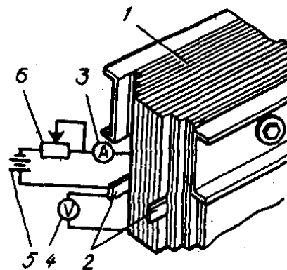
Рис. 20.4. Измерение сопротивления постоянному току межлистовой изоляции пакета магнитопровода:
