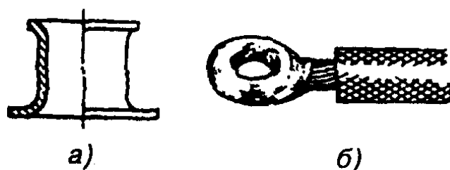
Рис. 2.13. Опрессовка многопроволочной медной жилы в кольцевом медном наконечнике:
