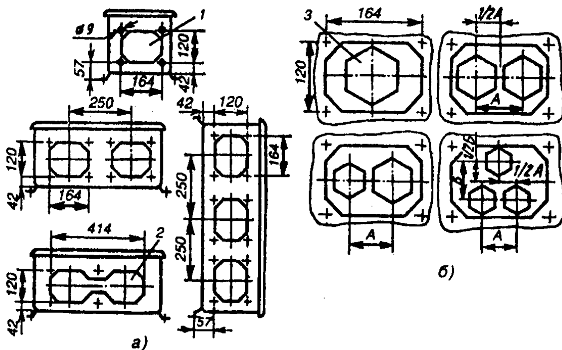
Рис. 6.5. Размеры и расположение соединительных окон проходными отверстиями ящиков РУС-Е:
