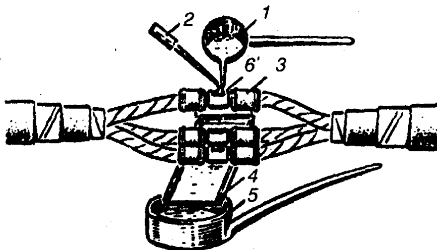
Рис. 2.15. Соединение жил способом полива расплавленным припоем:
