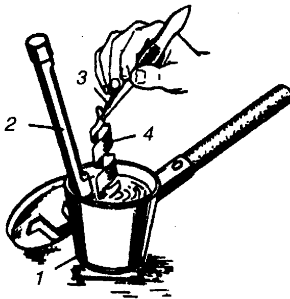
Рис. 7.12. Проверка бумажной изоляции кабеля на влажность:
