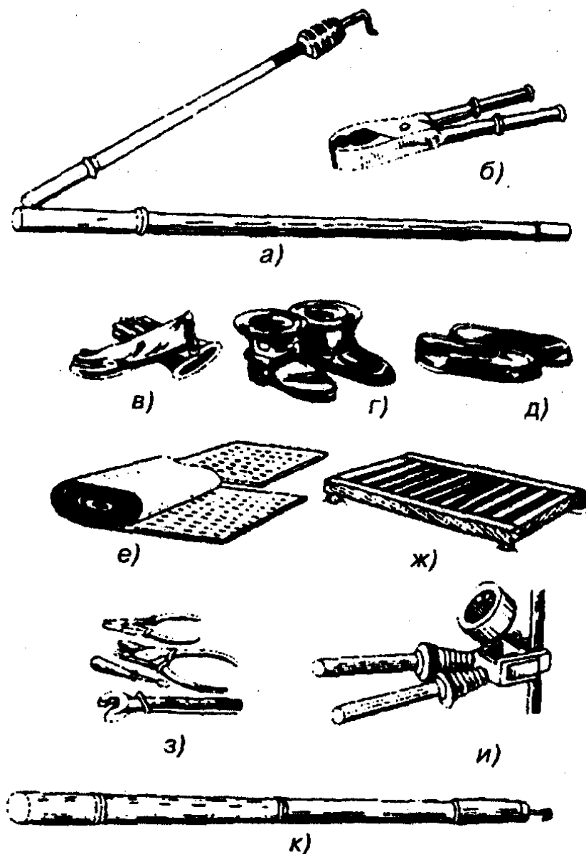
Рис. 22.4. Защитные средства:
