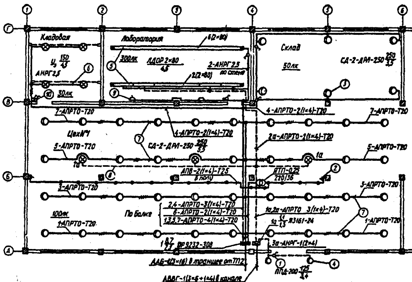
Рис. 1.9. План сети освещения
