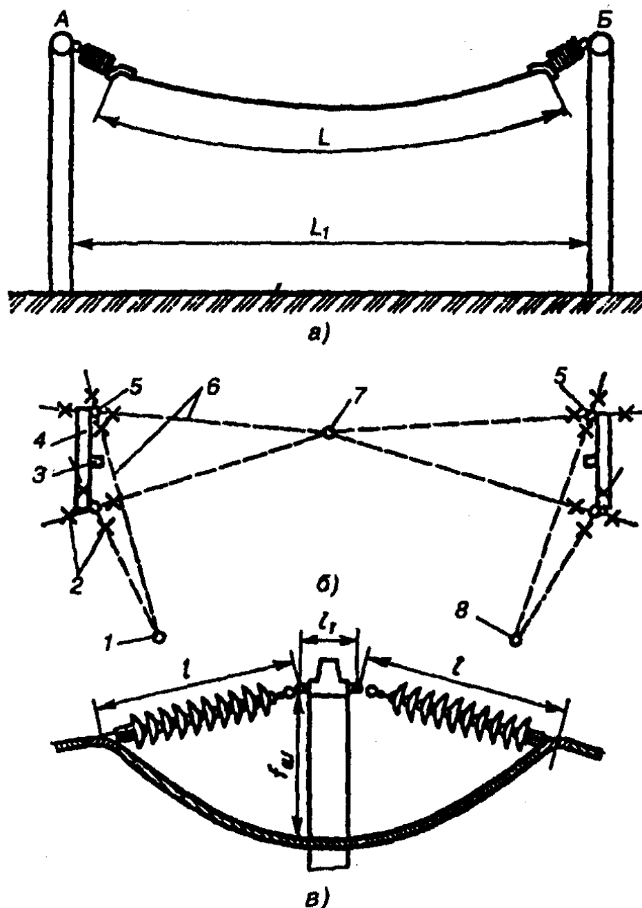
Рис. 11.4. Пролет ошиновки (а) и схема определения длин проводов в пролете (б) и шлейфе (в):
