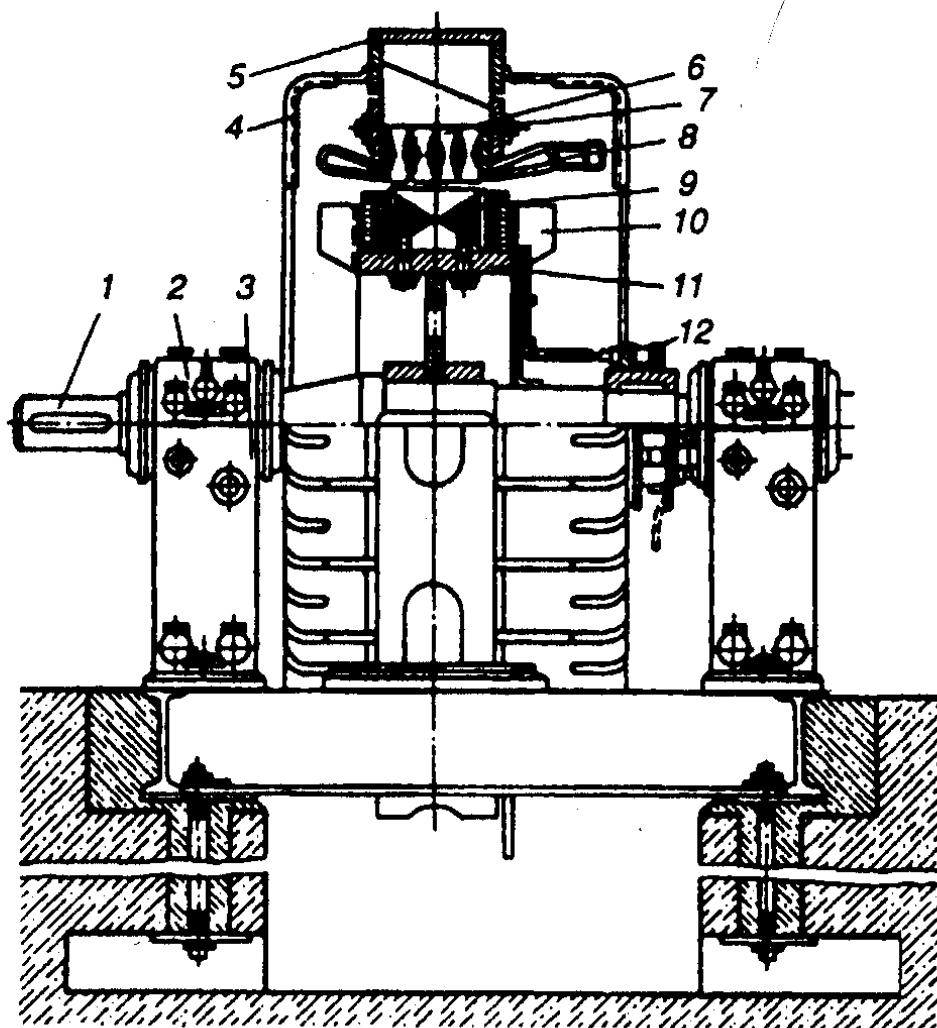
Рис. 12.3. Синхронный генератор:
