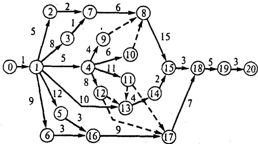
Рис. 1.11. Сетевой график проведения монтажных работ
