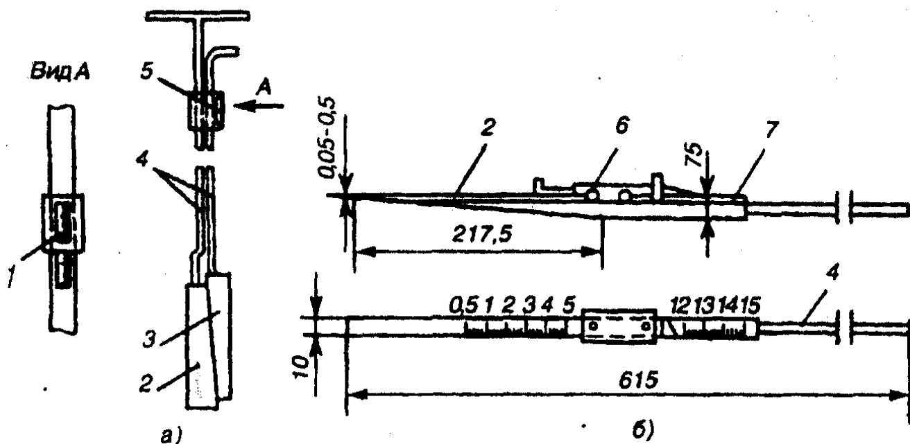
Рис. 12.13. Щупы:
