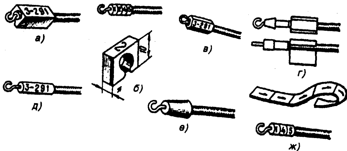
Рис. 9.8. Маркировочные бирки-оконцеватели:
