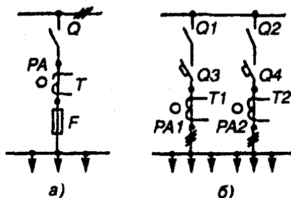
Рис. 6.3. Принципиальная схема линейной панели ПАР-11:
