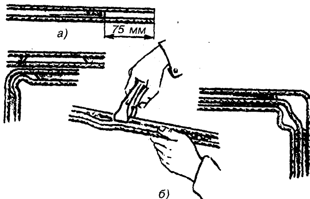
Рис. 4.3. Операции подготовки плоского провода перед монтажом:
