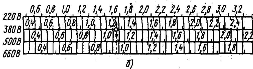
Рис. 20.19. Определение числа проводников в пазу при перемотке на другое напряжение (число параллельных проводников и ветвей не изменяется)
