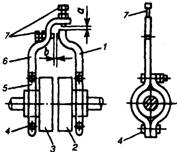
Рис. 12.8. Центровка валов с помощью радиально-осевых скоб:
