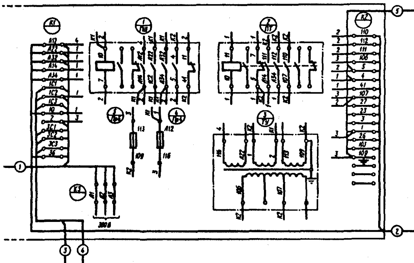
Рис. 1.6. Схема соединений, выполненная по адресной системе
