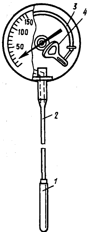
Рис. 17.3. Манометрический термометр:
