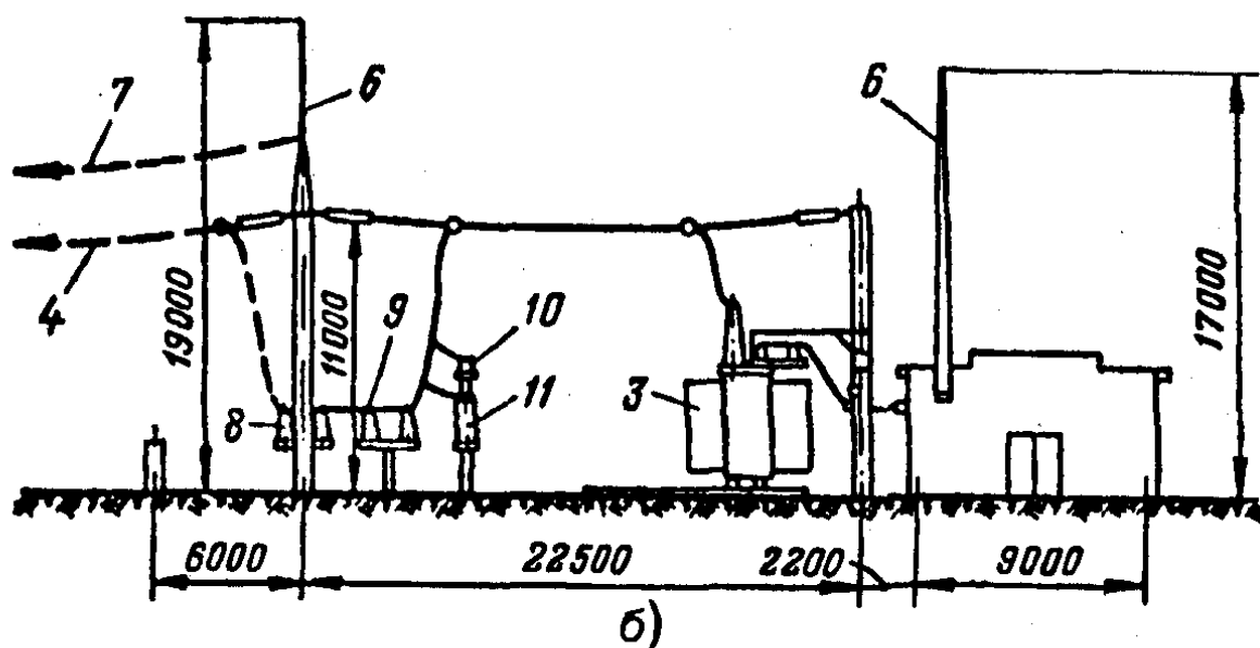
Рис. 11.1. План и разрез типовой ГПП 110/6-10 кВ с двумя трансформаторами мощностью 40 МВ · А:
