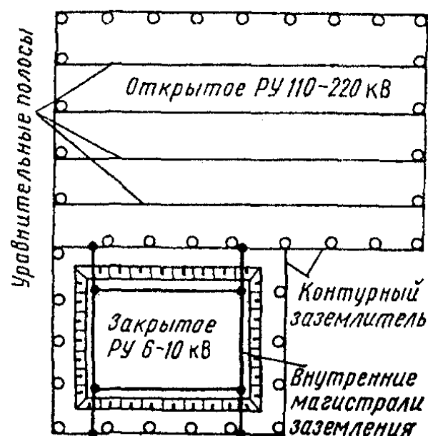
Рис. 3.2. Контур заземления подстанции
