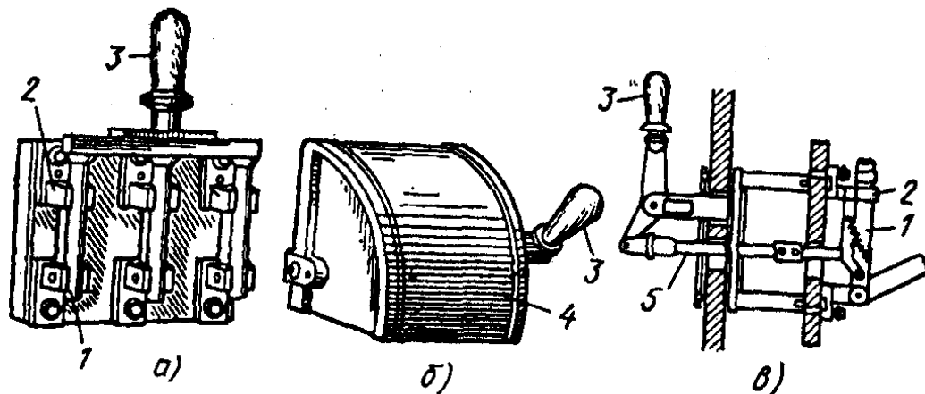
Рис. 20.29. Трехполюсный рубильник:
