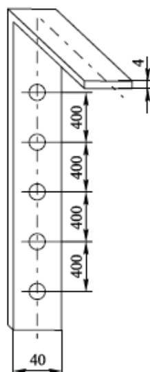
Рис. 11.12. Шаблон для разметки отверстий под крюки
