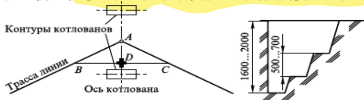
Рис. 11.8. Разбивка котлована под угловую анкерную опору (а) и форма котлована, отрытого вручную (б)
