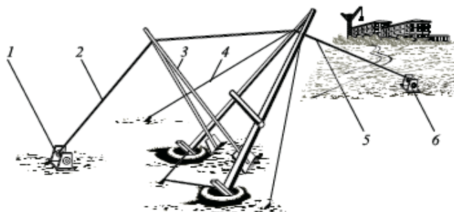
Рис. 11.14. Подъем и установка деревянной А-образной опоры с помощью лебедок и падающей стрелы:
