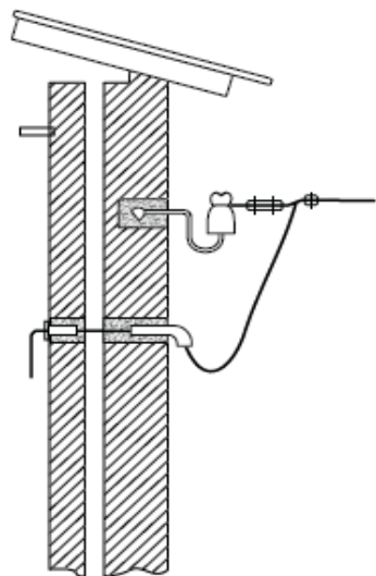
Рис. 11.29. Воздушный ввод в здание через стену
