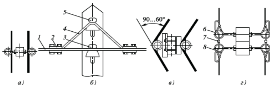
Рис. 11.27. Способы крепления проводов на изоляторах:
