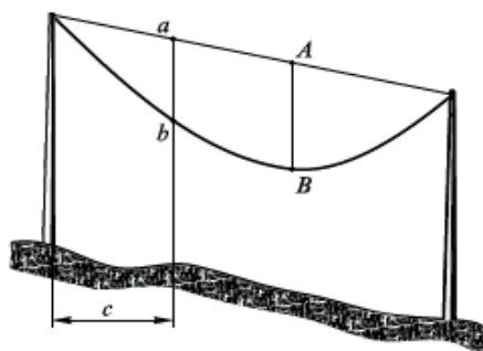
Рис. 11.25. Положение провода в пролете:
