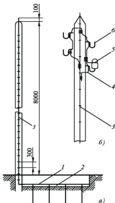
Рис. 11.28. Контур заземления на деревянной одностоечной опоре:
