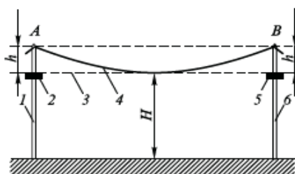
Рис. 11.26. Установка требуемой стрелы провеса методом визирования:
