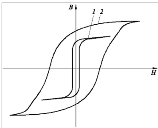
Рис. 5.13. Гистерезисные петли магнитомягкого 1 и магнитотвердого 2 материалов
