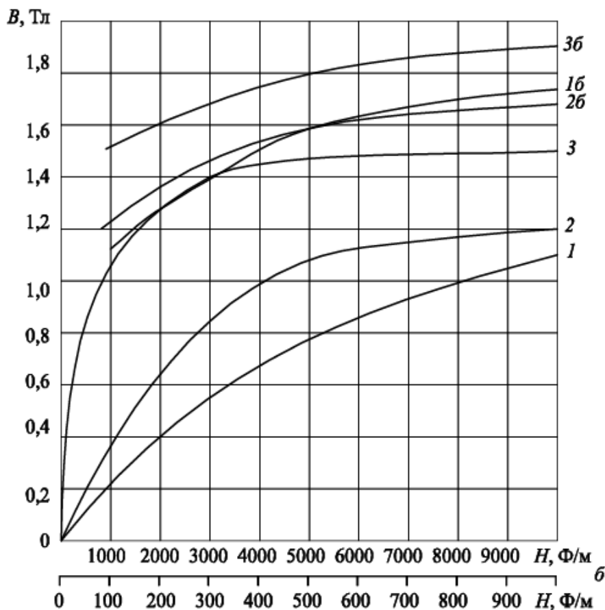
Рис. 5.12. Основные кривые намагничивания B(H) различных марок сталей: 1 – литая сталь; 2 – листовая электротехническая сталь 1512 (горячекатаная); 3 – листовая электротехническая сталь 3411 (холоднокатаная)
